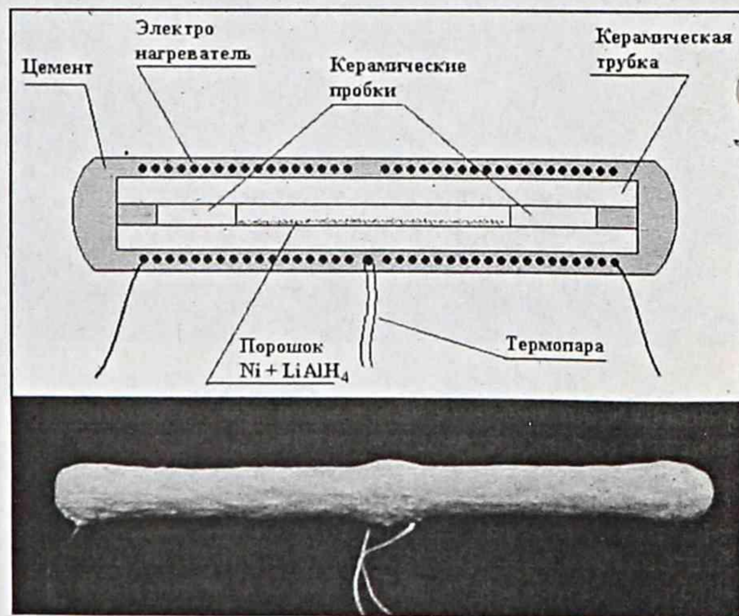
Трубка-реактор А.Пархомова
