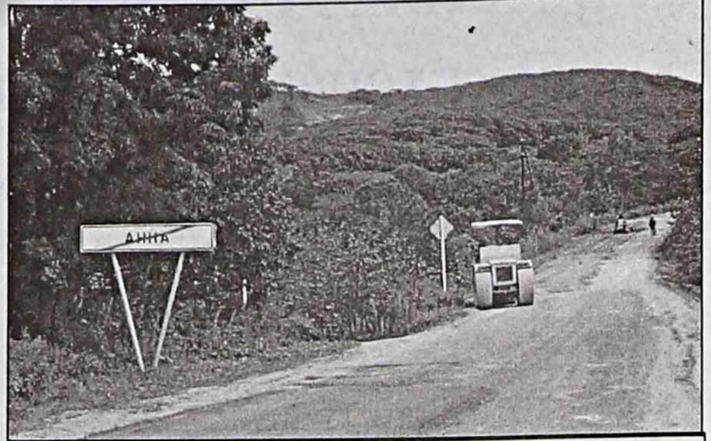
Подготовка дорожного полотна федеральной трассы Ливадия-Анна под асфальтирование
