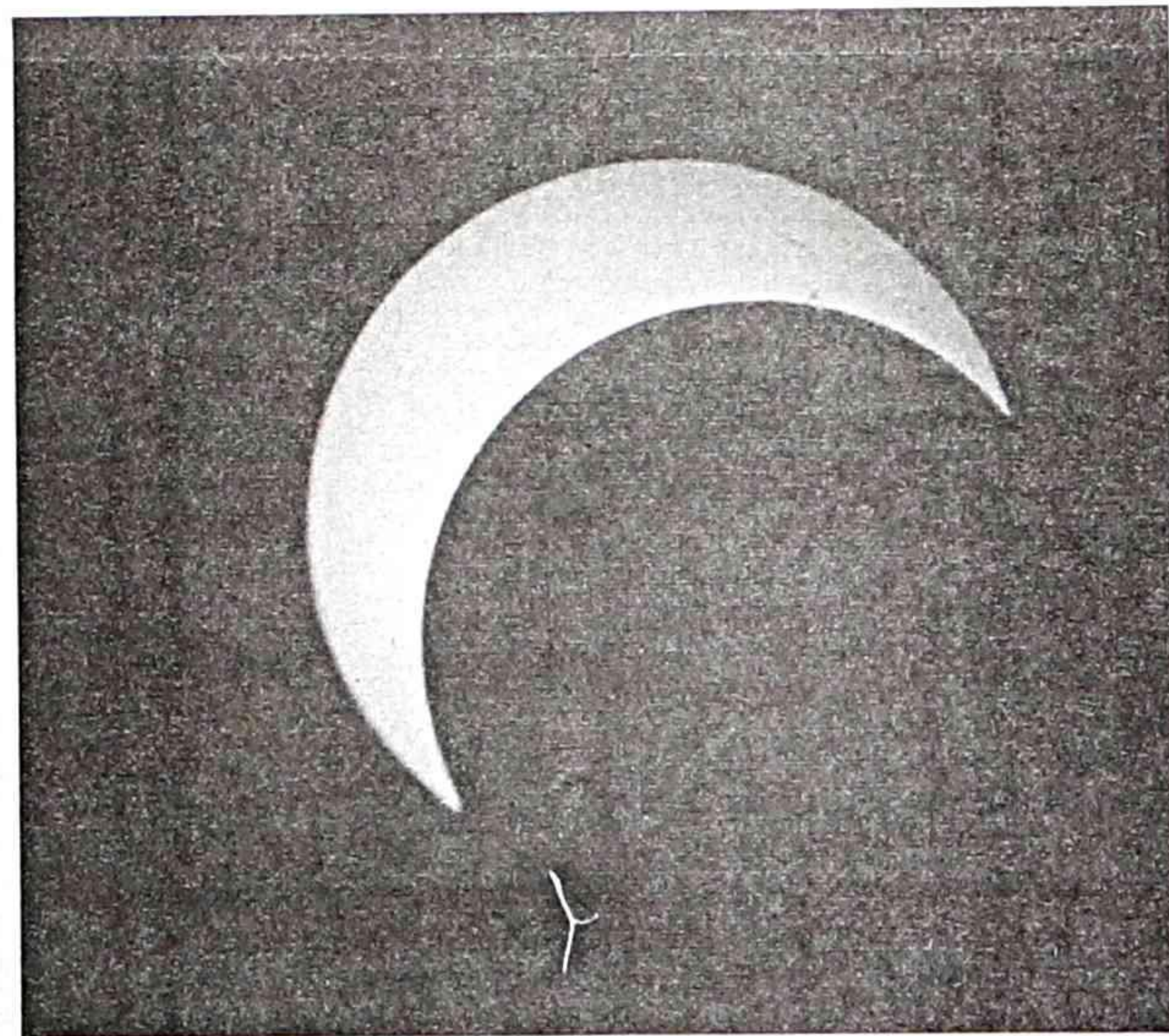
На фото максимальная стадия затмения (Солнце было закрыто Луной на 76%).
