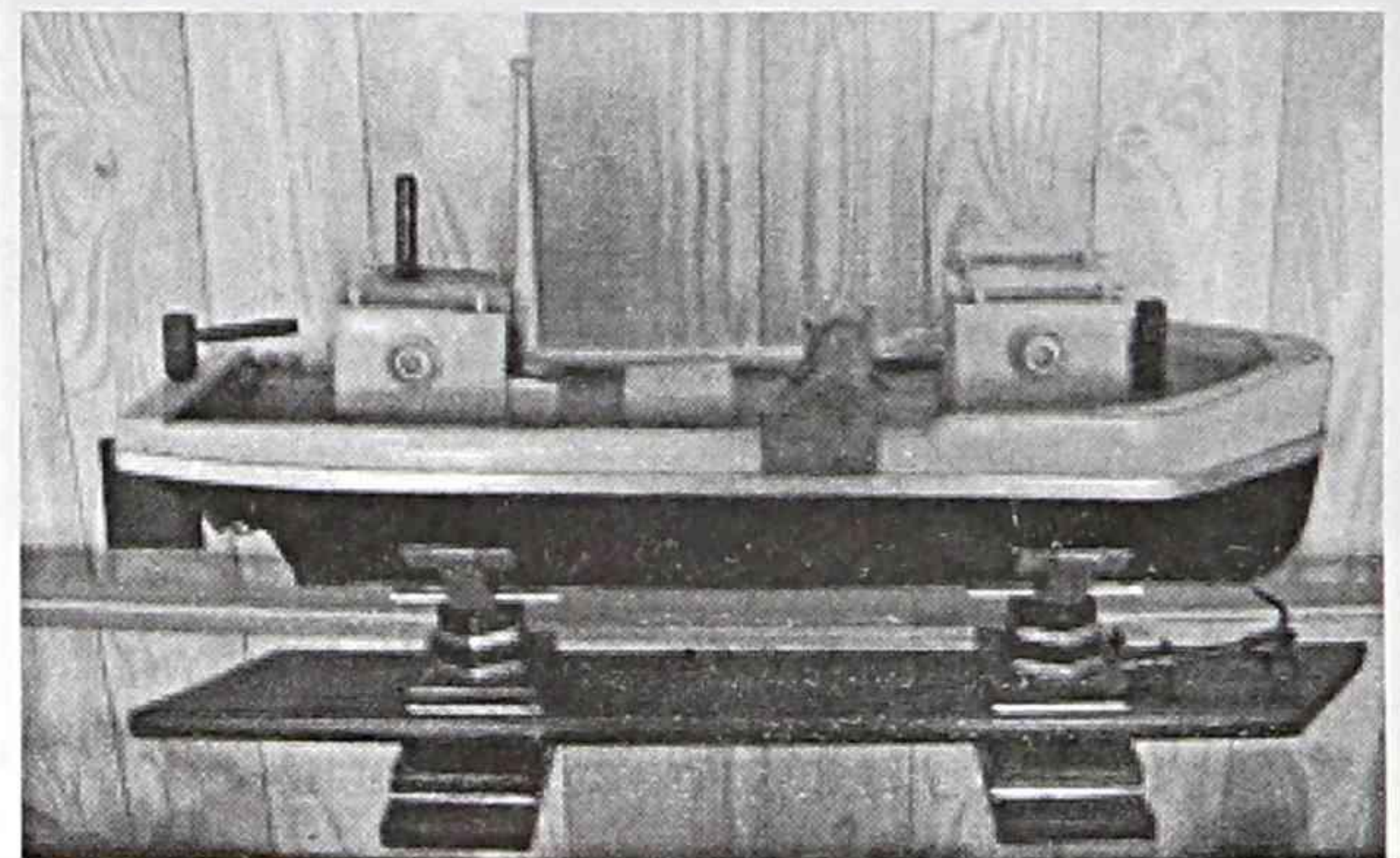
Судно типа Кавасаки - деревянное моторное судно для морского прибрежного промысла. Использовалось для лова рыбы, крабов и транспортировки кунгасов и шаланд в район промысла (к ставным неводам).
